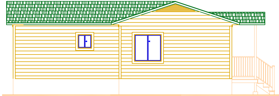
GEMDUS-4 Right Elevation
